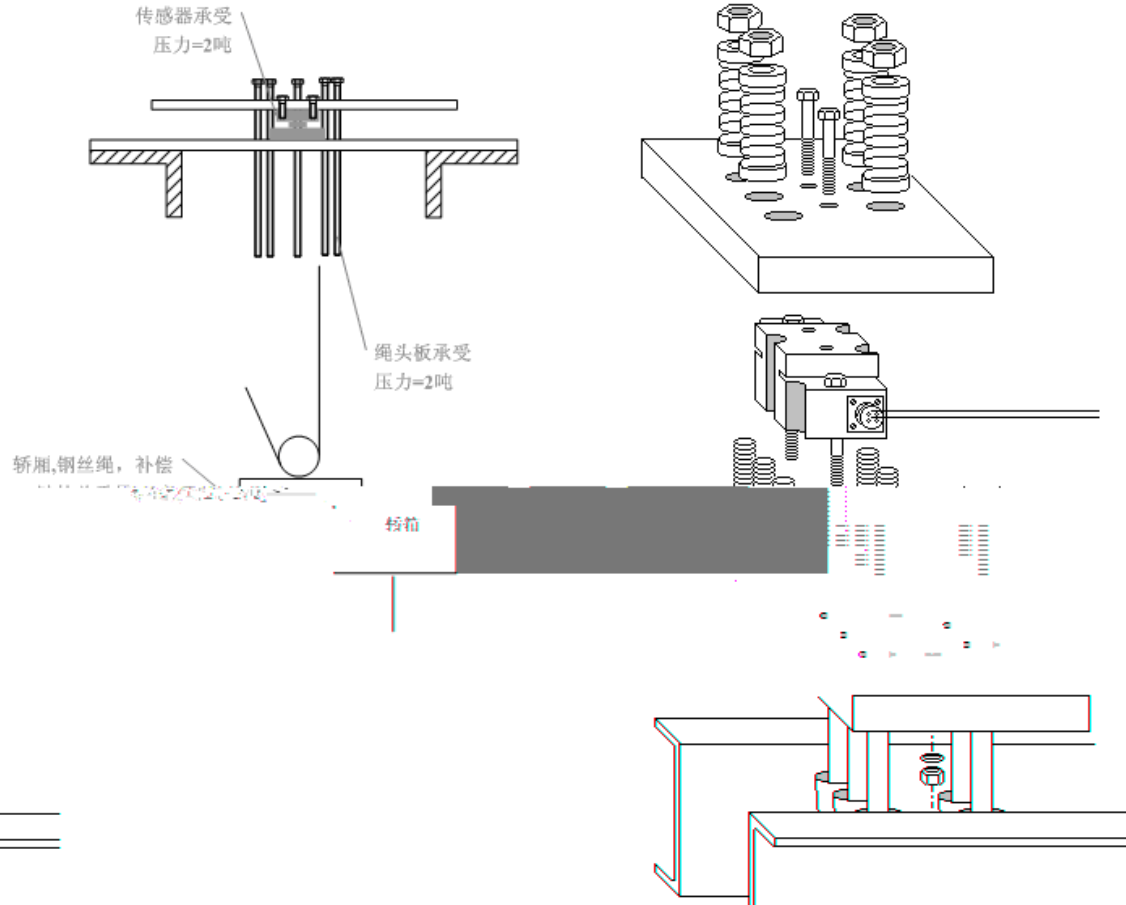
传感器安装方式（不带支架）
